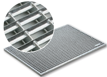
Maschenrost mit V-Stab Stahl verzinkt, Maschenweite ca. 9/31 mm.
