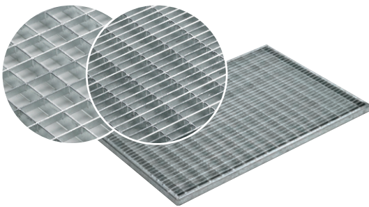
Maschenroste Maschenweite 30/30 und 30/10, Stahl verzinkt
